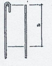
2.3 ระยะเวลาการเชื่อมเหล็ก (STANDARD HOOK)
