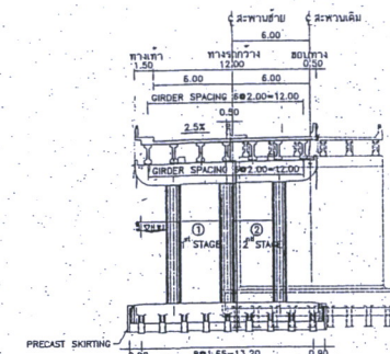
รูปตัดความกว้างดอมกลางน้ำ ช่วง 30.00 ม. ขนาดกว้าง 1:200
