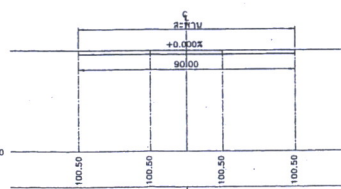
รูปตัดแสดงระดับหลังทางจากปลายสะพาน ขนาดกว้าง 1:500 , มุม 1:1,000
