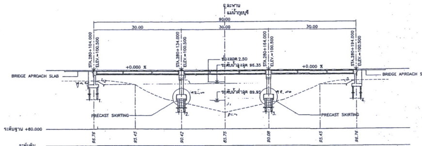
รูปตัดที่ ๑ สะพานด้านซ้ายทาง ขนาดกว้าง 1:400
