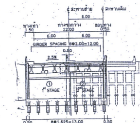
รูปตัดความกว้างดอมริมฝั่ง ช่วง 30.00 ม. ขนาดกว้าง 1:200
