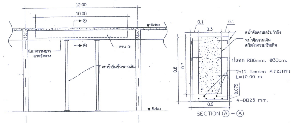
แบบซ่อมแซมและเสริมกำลังรูปแบบที่ 2
