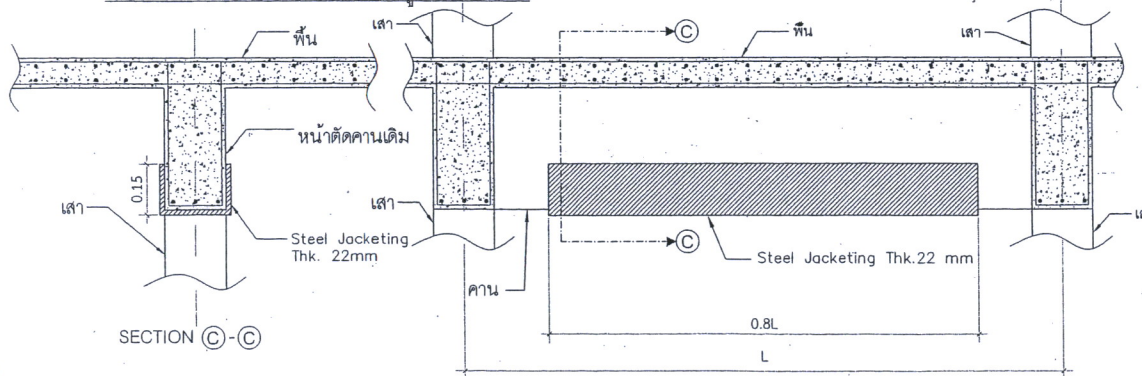
แบบซ่อมแซมและเสริมกำลังรูปแบบที่ 5
