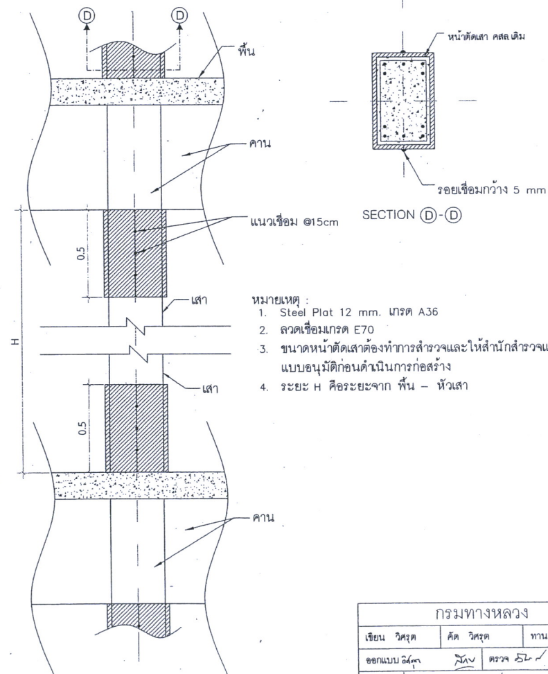
แบบซ่อมแซมและเสริมกำลังรูปแบบที่ 4
