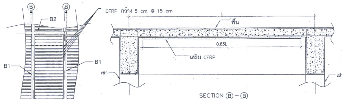
แบบซ่อมแซมและเสริมกำลังรูปแบบที่ 3
