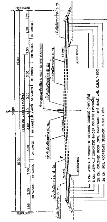
รูปตัดถนน C
