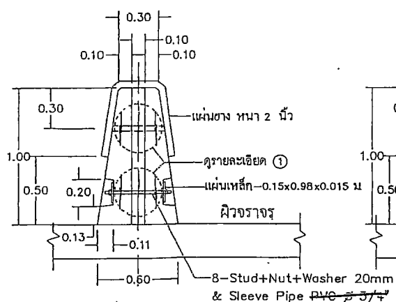
รูปตัด A SHEAR KEY
