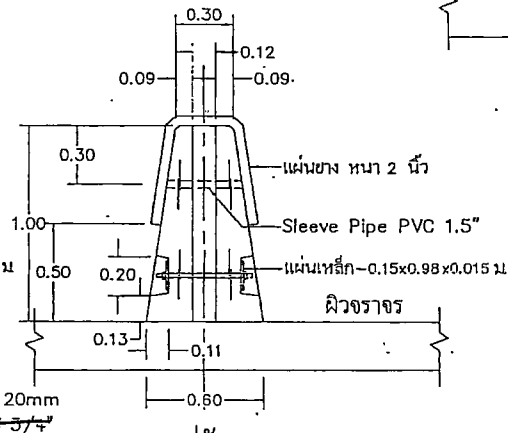
รูปตัด B / SHEAR KEY
