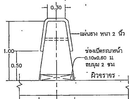
รูปตัด C
