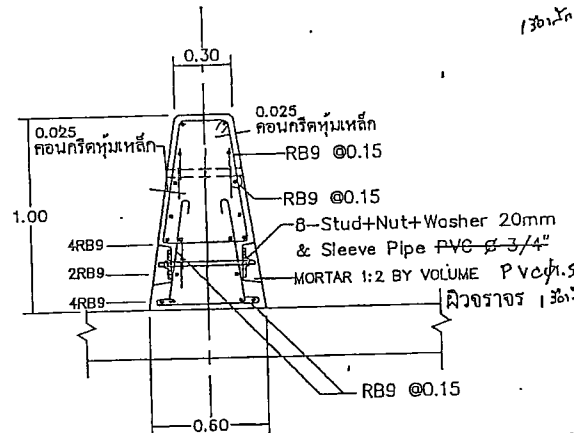
รายละเอียดเหล็กเสริม
