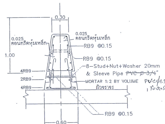
รายละเอียดหลักเสริม
