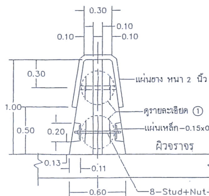
รูปตัด A SHEAR KEY
