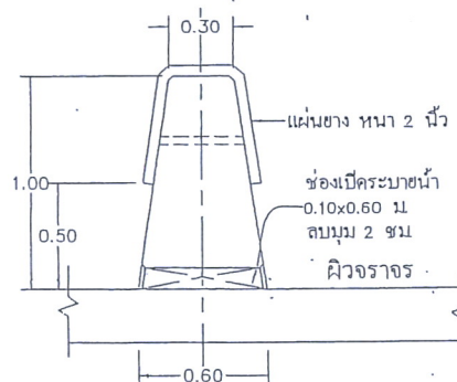
รูปตัด C
