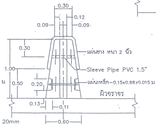
รูปตัด B SHEAR KEY
