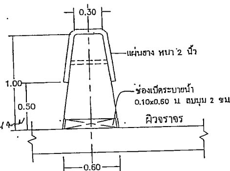
รูปตัด C
