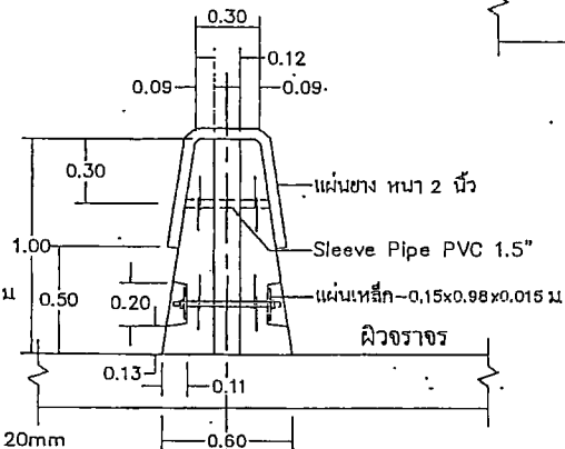
รูปตัด B
