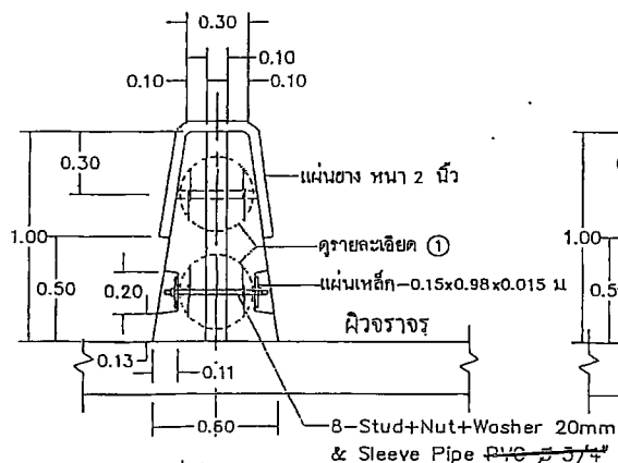
รูปตัด A
