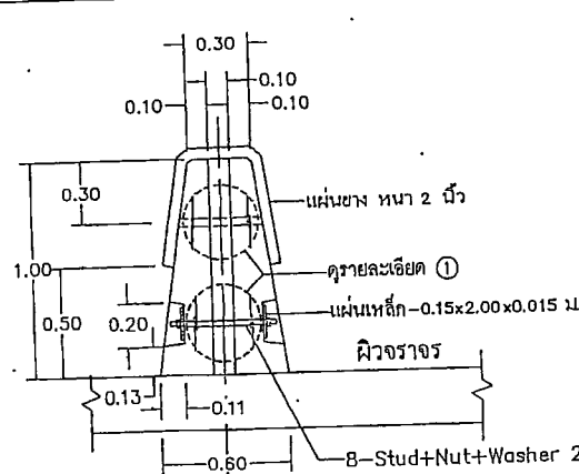
รูปตัด A
