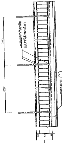
แบบขยายโครงสร้างหลังคา (กรณีติดตั้งตามแบบเดิมกับรางเดิม)
